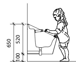
Attentes plomberie
